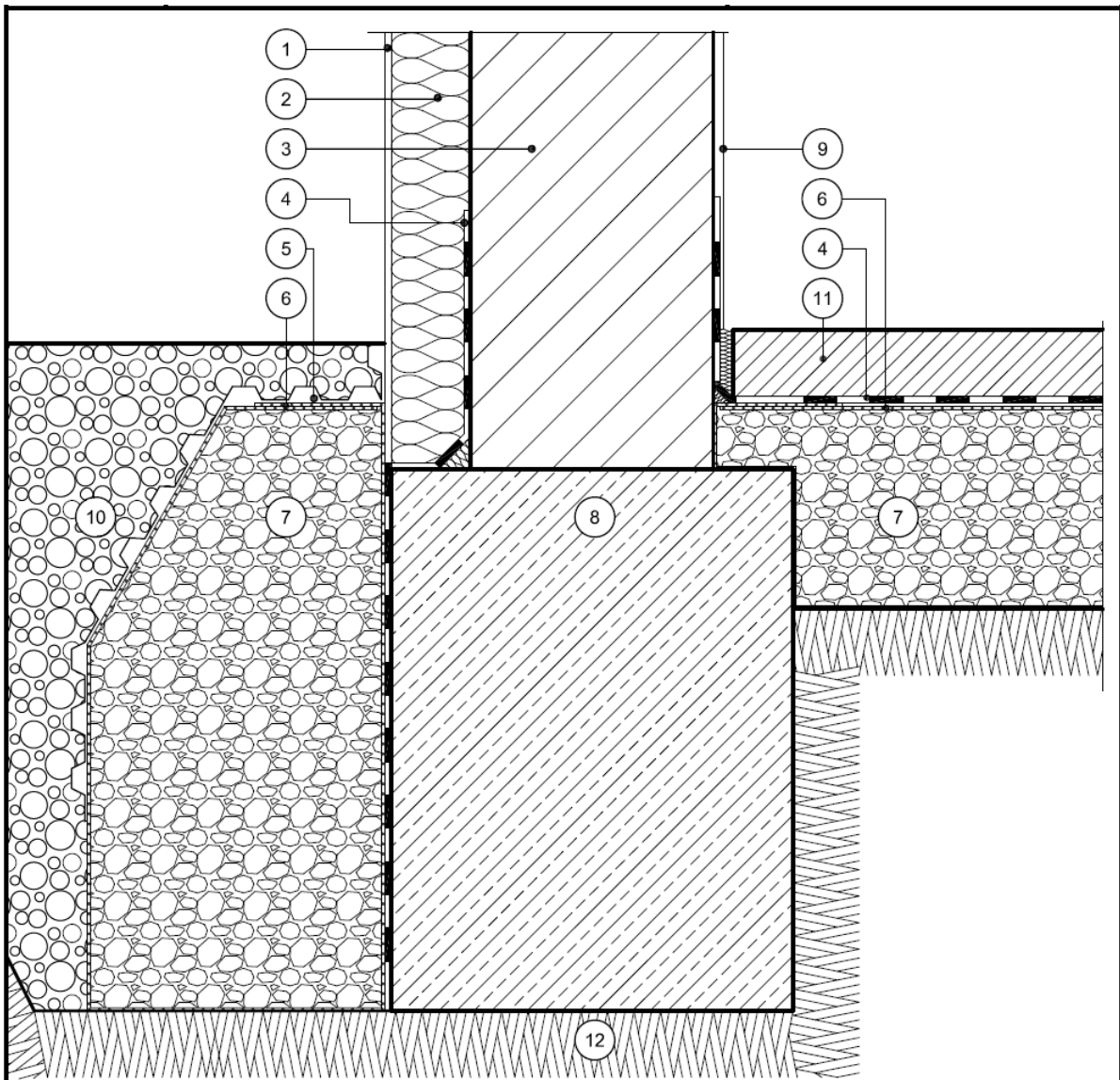
Vertikalschnitt
